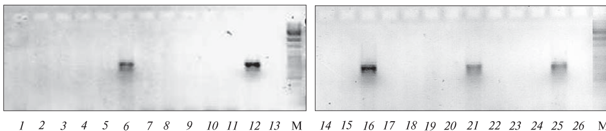
Рис. 2. Електрофореграма продуктів ампліфікації локусу sms-S у лінії кукурудзи W8 (1), W8Т (2), W8М (3), W8Б (4), W8С (5), W8МВ (6), W8ТВБ (7), W8БТВ (8), W8БВ (9), P502 (10), P502Т (11), P502М (12), P502С (13), P502ТВ (14), P502МВ (15), P502БВ (16), P502ТВБ (17), P502БТВ (18), СК32 (19), СК32Т (20), СК32М (21), СК32Б (22), СК32С (23), СК32ТВ (24), СК32БВ (25). М – маркер молекулярної маси GeneRuler 100 bp DNA Ladder Plus
